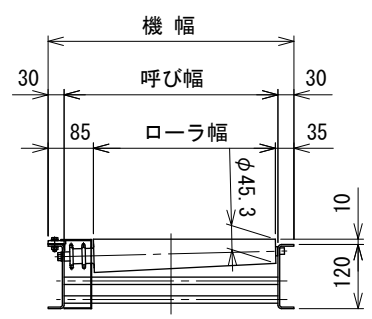
△ 一般断面図
