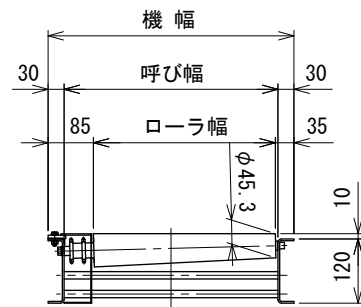
① 一般断面図
