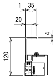
A-A 矢視図
