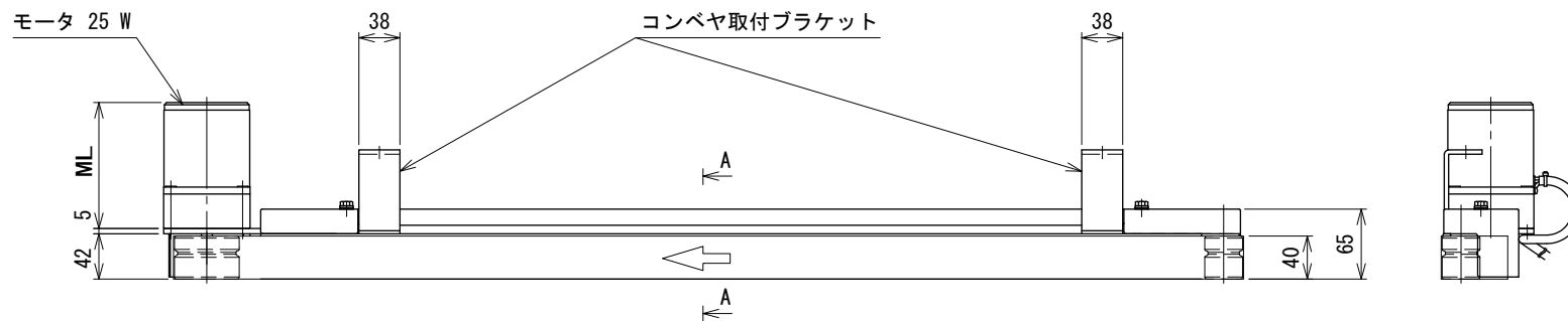
モータ寸法表 ML (mm)
